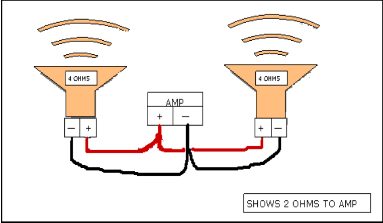
PARALLELL WIRING
